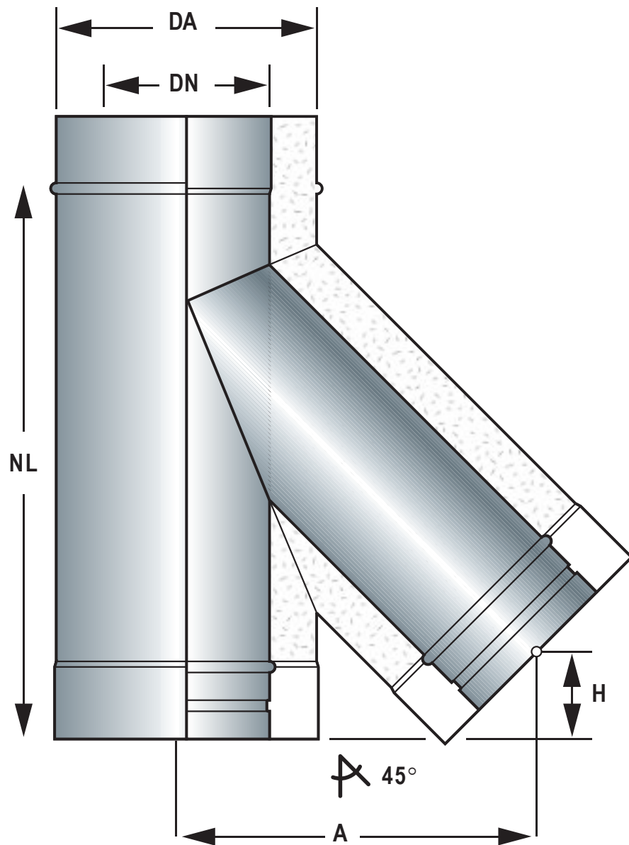
F-Anschluss 45° mit Kondensatabweiser
