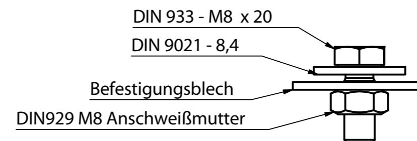
Befestigungsblech (1:1)
