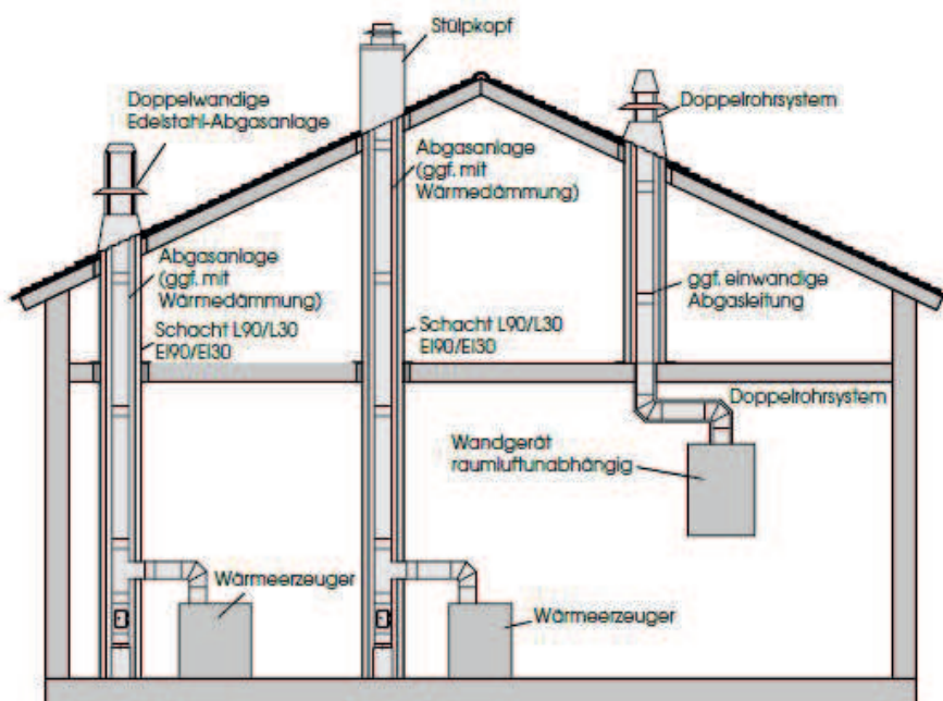
Beispiel verschiedene Aufbauarten (Systemwechsel, Stülpkopf, Deckenmontage)
